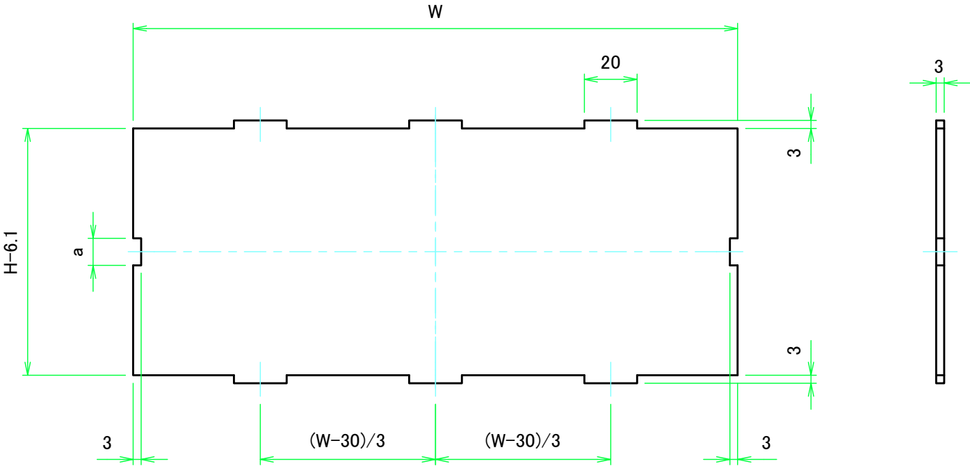
Wパネル1表面 / W panel 1 Frontside
